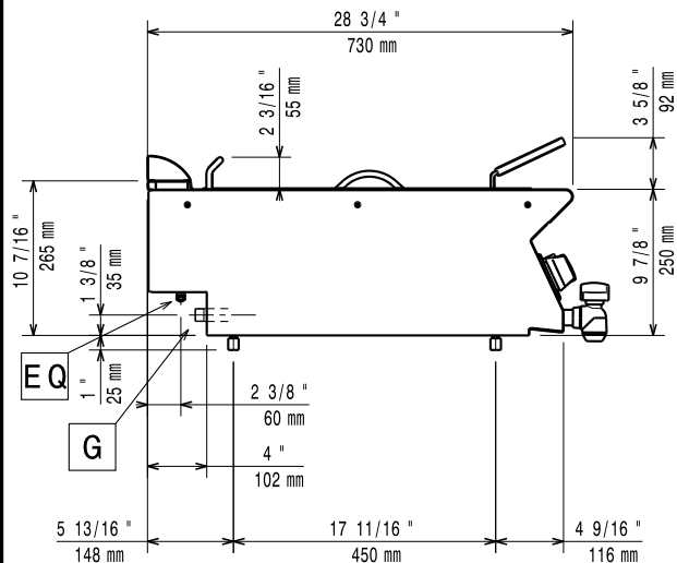
Oldalnézet
